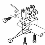
Fig. 555A DIAMETRI - DIAMETERS DIAMETRES Y= 28mm : Kit n° T-8117-C Y= 30mm : Kit n° T-8117-C1 Y= 32mm : Kit n° T-8117-C2
