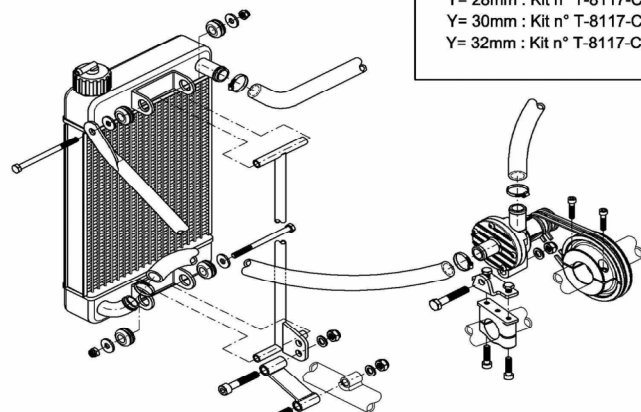
SCHEMA DI MONTAGGIO ASSEMBLING LAYOUT SCHEMA DE MONTAGE
